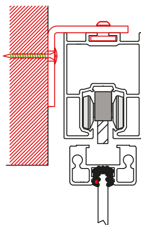
APPLICAZIONE STANDARD
