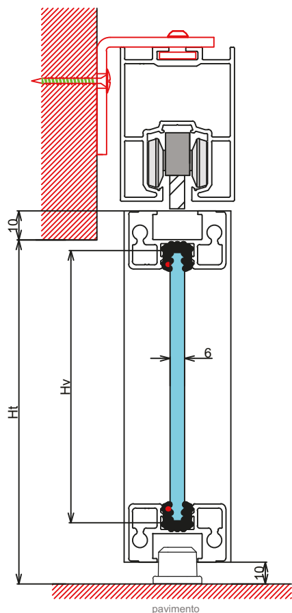
DIMENSIONAMENTO ANTA
