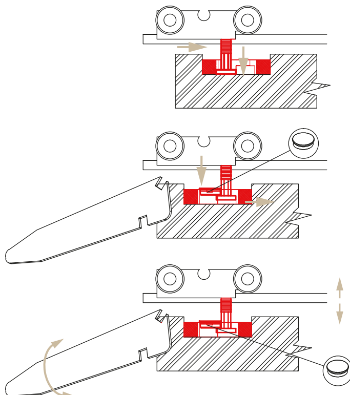
DETTAGLIO AGGANCIAMENTO PORTA-SISTEMA AMMORTIZZATO
