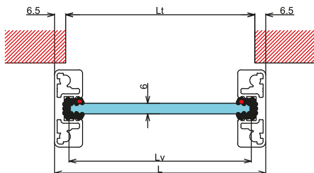
DIMENSIONAMENTO ORIZZONTALE
