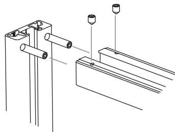
DETTAGLIO AGGANCIAMENTO PORTA-SISTEMA AMMORTIZZATO
