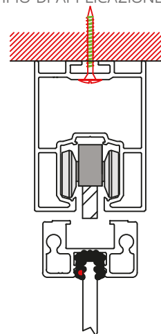
LAVORAZIONE DI FORATURA GUIDA PER FISSAGGIO A SOFFITTO DA RICHIEDERE SPECIFICAMENTE.
