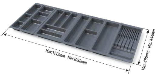
105-83-26 120 'lik Modül for module 120
