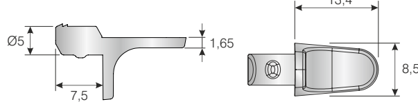
Ahşap için For wood
