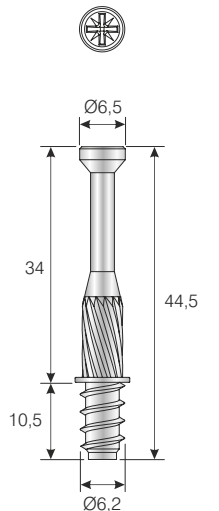
Pozidriv PZ2 Philips PH2
