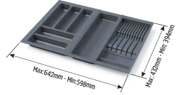
105-45-27 70 'lik Modül for module 70
