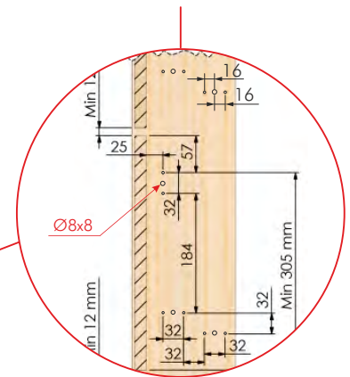
A-A VIEW
