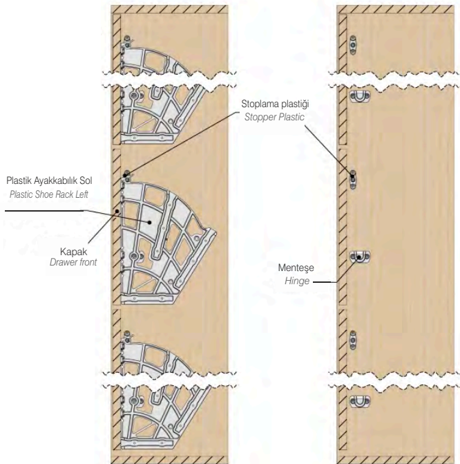
A-A VIEW
