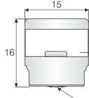
M10 Metal Setskur M10 Metal Screw
