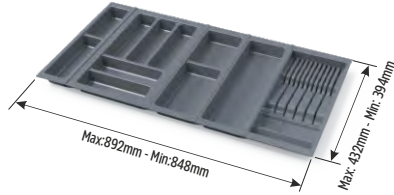
105-45-32 95 'lik Modül for module 95
