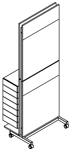
S-2015 METAL STRUCTURE 4 PANELS + SHELF ESTRUCTURA PARA 4 PANELES S-2015 + 1 REPISA
