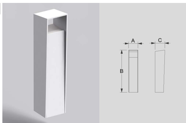
A: 330 mm B: 1500 mm C: 345 mm
