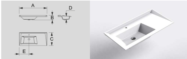
A: 1004 mm B: 169 mm C: 480 mm Available with ØØ D: 110 mm E: 350 mm Disponible en ØØ.
