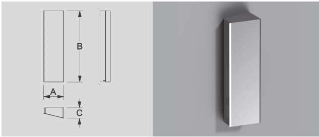
A: 423 mm B: 1500 mm C: 270 mm
