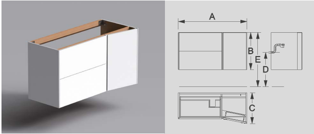
A: 1100 mm B: 595 mm C: 488 mm D: 550 mm E: 870 mm
