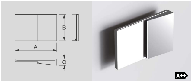
A: 910-1105 mm B: 700 mm C: 170 mm
