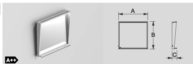
A: 700 mm B: 666 mm C: 118 mm
