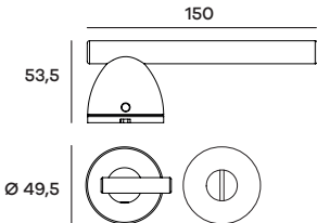
BLORO24W29 Maniglia su rosetta WC Doorhandle on WC rose
