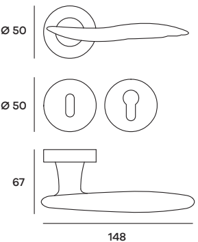
FLYRO09P (Patent) FLYRO09Y (Yale) Maniglia su rosetta Doorhandle on rose
