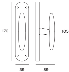
SABMTRC02 Maniglia per cremonese Windowhandle
