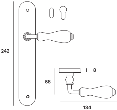
OTTPL02P (Patent) OTTPL02Y (Yale) Maniglia su placca Doorhandle on plate
