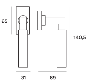
INFDK03 Maniglia per finestra DK Windowhandle DK
