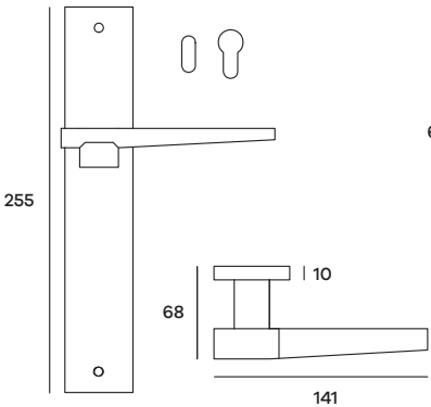
VETPL59P (Patent) VETPL59Y (Yale) Maniglia su placca Doorhandle on plate
