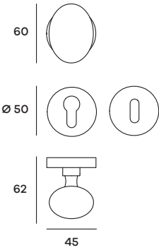
OVARO06P (Patent) OVARO06Y (Yale) Maniglia su rosetta Doorhandle on rose
