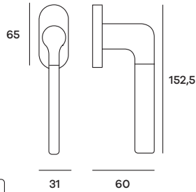
LINDK01 Maniglia per finestra DK Windowhandle DK
