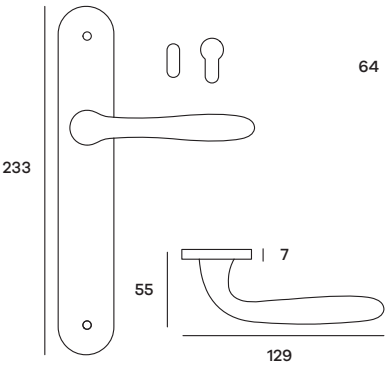
GOCPL15P (Patent) GOCPL15Y (Yale) Maniglia su placca Doorhandle on plate
