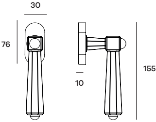
OCTDK01 Maniglia per finestra DK Windowhandle DK
