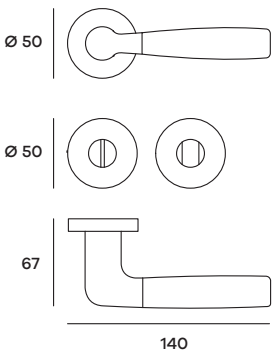
JETRO02W01 Maniglia su rosetta WC Doorhandle on WC rose
