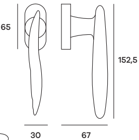
FLYDK01 Maniglia per finestra DK Windowhandle DK
