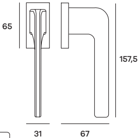
SIMDK03 Maniglia per finestra DK Windowhandle DK
