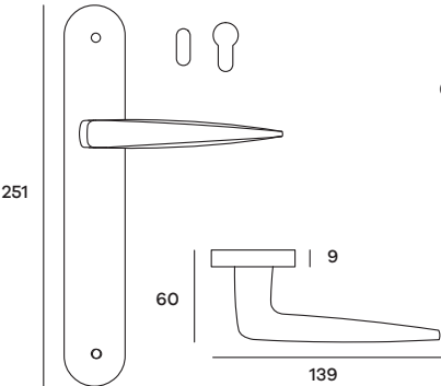
MIAPL05P (Patent) MIAPL05Y (Yale) Maniglia su placca Doorhandle on plate
