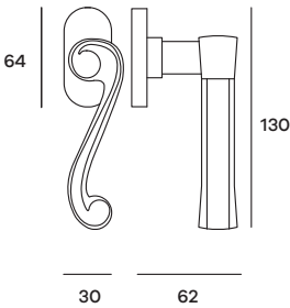
RICDK01 Maniglia per finestra DK Windowhandle DK
