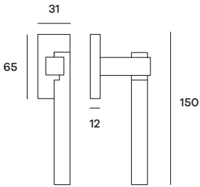
CODDK03 Maniglia per finestra DK Windowhandle DK
