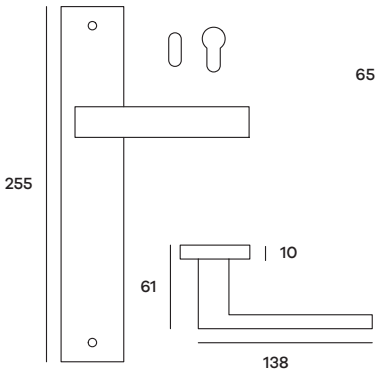
BILPL59P (Patent) BILPL59Y (Yale) Maniglia su placca Doorhandle on plate
