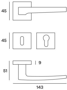
SYDRO57P (Patent) SYDRO57Y (Yale) Maniglia su rosetta Doorhandle on rose
