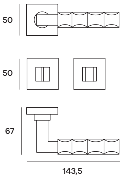
SNARO53W07 Maniglia su rosetta WC Doorhandle on WC rose
