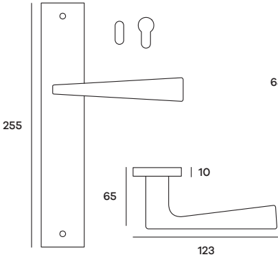
KUBPL59P (Patent) KUBPL59Y (Yale) Maniglia su placca Doorhandle on plate
