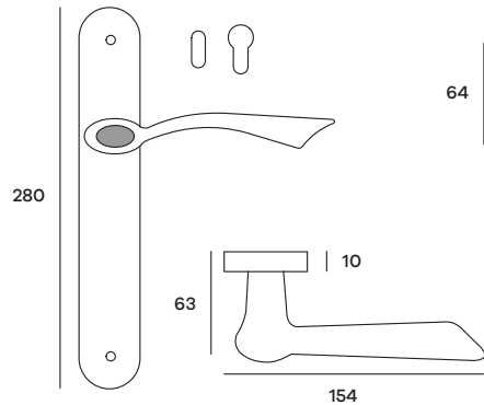
HELPL01P (Patent) HELPL01Y (Yale) Maniglia su placca Doorhandle on plate
