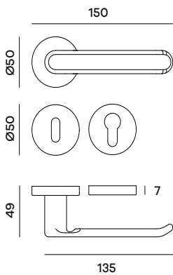
TEORO02P (Patent) TEORO02Y (Yale) Maniglia su rosetta Doorhandle on rose
