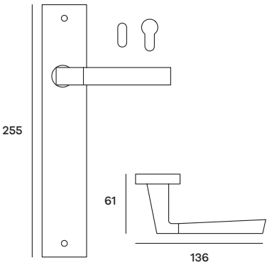
EASPL59P (Patent) EASPL59Y (Yale) Maniglia su placca Doorhandle on plate
