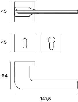
SIXRO85P (Patent) SIXRO85Y (Yale) Maniglia su rosetta Doorhandle on rose
