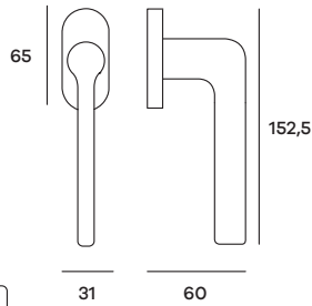
LINDK01 Maniglia per finestra DK Windowhandle DK
