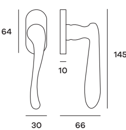
ASIDK01 Maniglia per finestra DK Windowhandle DK
