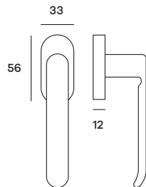
TEODK01 Maniglia per finestra DK Windowhandle DK
