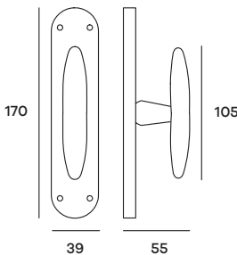
FUTMRTCRO2 Maniglia per cremonese Windowhandle
