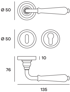
CLARO07P (Patent) CLARO07 (Yale) Maniglia su rosetta Doorhandle on rose
