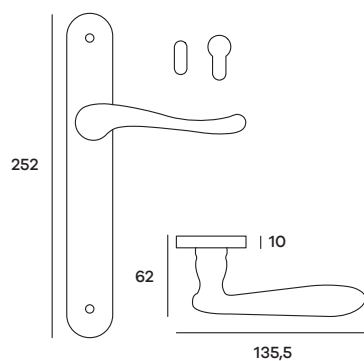
ASIPLO2P (Patent) ASIPLO2Y (Yale) Maniglia su placca Doorhandle on plate
