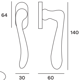
VERDK01 Maniglia per finestra DK Windowhandle DK
