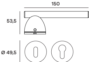
BLORO24P (Patent) BLORO24Y (Yale) Maniglia su rosetta Doorhandle on rose
