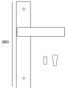
PNTPL59P (Patent) PNTPL59Y (Yale) Maniglia su placca Doorhandle on plate
