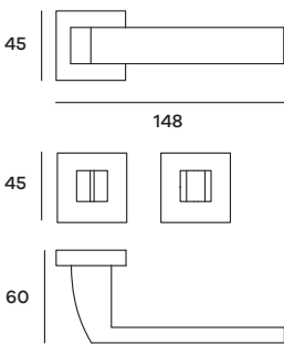
GENRO52W07 Maniglia su rosetta WC Doorhandle on WC rose
