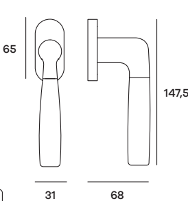
JETDK01 Maniglia per finestra DK Windowhandle DK
