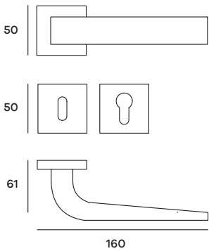
NAVRO52P (Patent) NAVRO52Y (Yale) Maniglia su rosetta Doorhandle on rose
