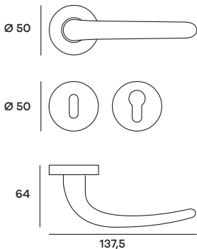
SABRO02P (Patent) SABRO02Y (Yale) Maniglia su rosetta Doorhandle on rose
