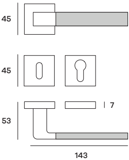
BIBRO57P (Patent) BIBRO57Y (Yale) Maniglia su rosetta Doorhandle on rose
