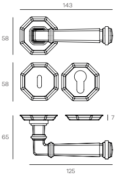
DMTRO85P (Patent) DMTRO85Y (Yale) Maniglia su rosetta Doorhandle on rose
