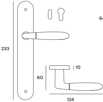
DROPL15P (Patent) DROPL15Y (Yale) Maniglia su placca Doorhandle on plate
