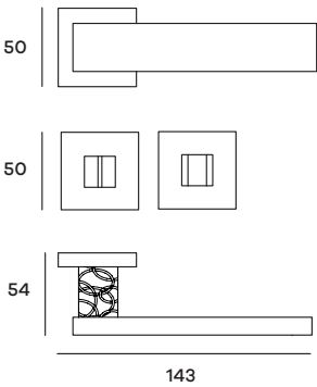
MUSRO72W01 Maniglia su rosetta WC Doorhandle on WC rose
