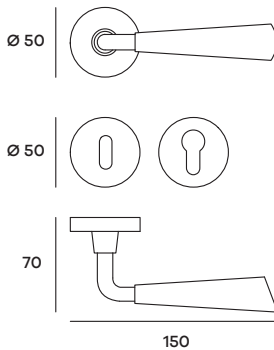
NILRO24P (Patent) NILRO24Y (Yale) Maniglia su rosetta Doorhandle on rose
