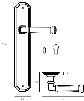
DMTPL84P (Patent) DMTPL84Y (Yale) Maniglia su placca Doorhandle on plate
