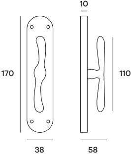
ASIMRTR02 Maniglia per cremonese Windowhandle
