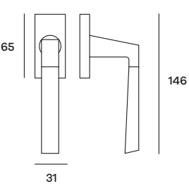
EASDK03 Maniglia per finestra DK Windowhandle DK
