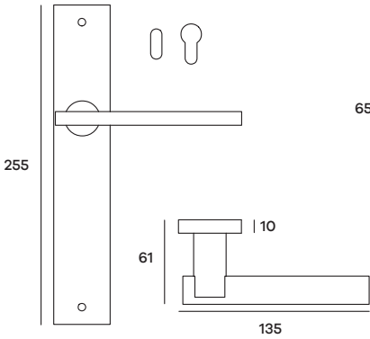
SQUPL59P (Patent) SQUPL59Y (Yale) Maniglia su placca Doorhandle on plate
