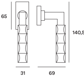
SNADK03 Maniglia per finestra DK Windowhandle DK
