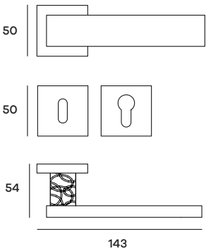
MUSRO72P (Patent) MUSRO72Y (Yale) Maniglia su rosetta Doorhandle on rose
