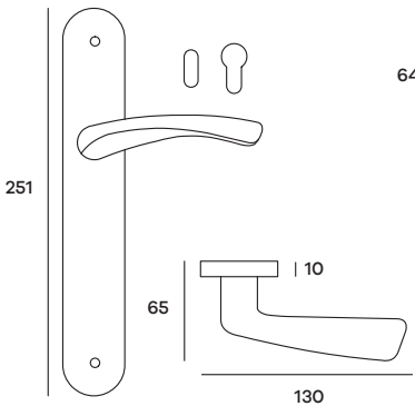
GALPL05P (Patent) GALPL05Y (Yale) Maniglia su placca Doorhandle on plate
