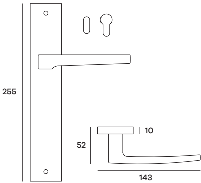
SYDPL59P (Patent) SYDPL59Y (Yale) Maniglia su placca Doorhandle on plate
