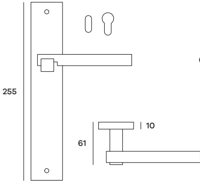
CODPL59P (Patent) CODPL59Y (Yale) Maniglia su placca Doorhandle on plate
