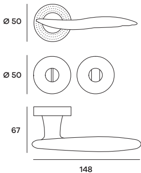
FLYRO15W01 Maniglia su rosetta WC Doorhandle on WC rose
