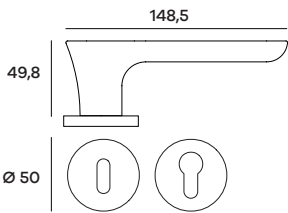
PNTRO54P (Patent) PNTRO54Y (Yale) Maniglia su rosetta Doorhandle on rose
