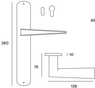
WOOPL05P (Patent) WOOPL05Y (Yale) Maniglia su placca Doorhandle on plate
