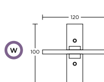
ΓΡΥΛΟΧΕΡΟ WINDOW HANDLE
