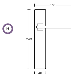
ΧΕΙΡΟΛΑΒΗ ΠΛΑΚΑ PLATE HANDLE
