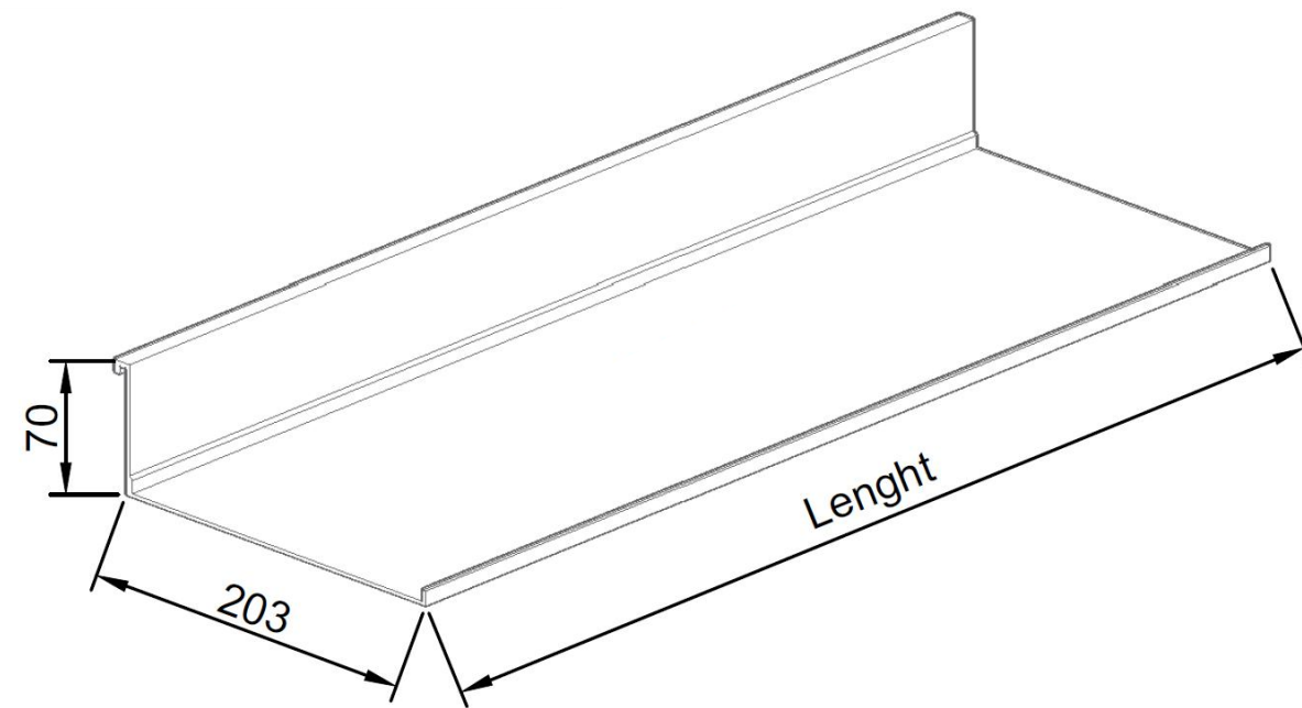
• Aluminium Shelf Dimensions
